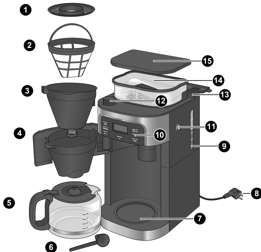
Abb. 1: Parti dell'apparecchio
