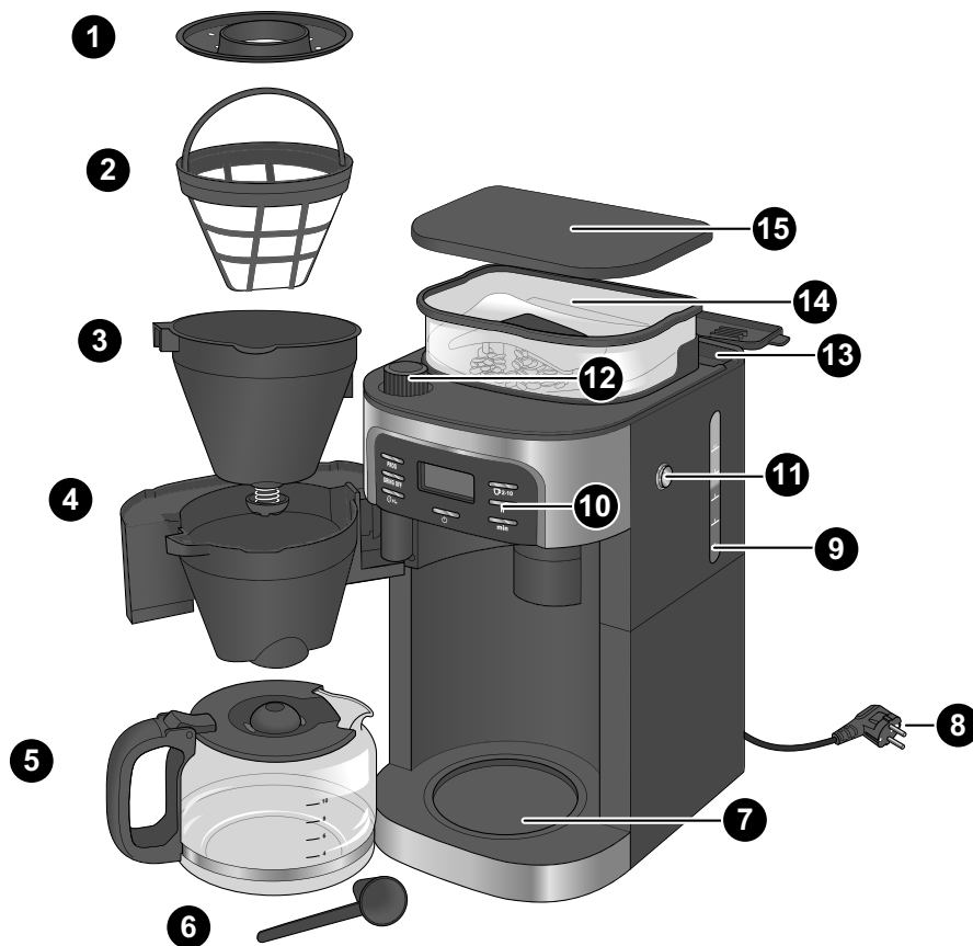
Abb. 1: Partes del aparato
